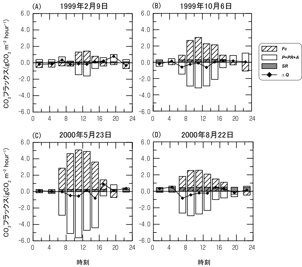
図 5.1.6 森林大気の CO 2 収支の計算結果 (小栗・檜山, 2002)
